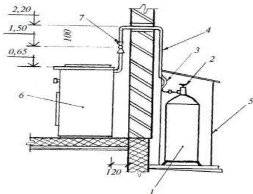
Рис. 78. Установка баллона со сжиженным газом вне дома:
